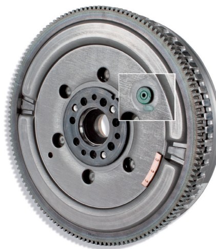
Figura 1: Con el primer arranque, el seguro de transporte se rompe en el interior del volante bimasa
