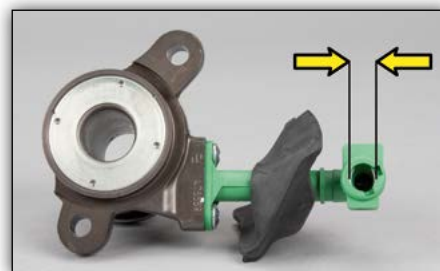
4. ábra: LuK CSC 510 0137 10 Hidraulikacsatlakozás 12,2 mm
