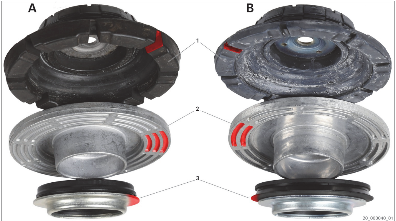
Sl. 1: Potporni ležaj opružne noge - varijanta A/B
