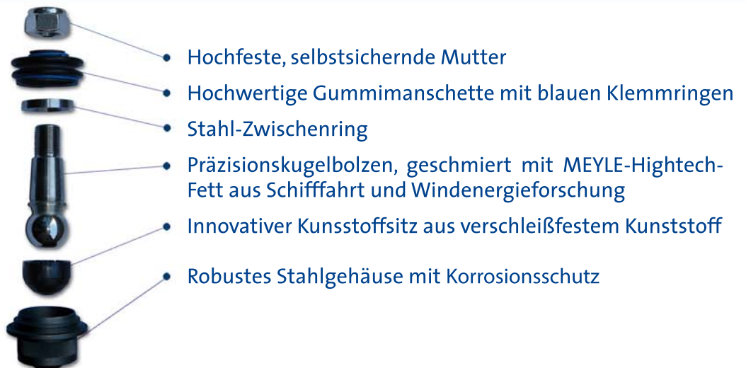
Explosionsgrafik Traggelenk
