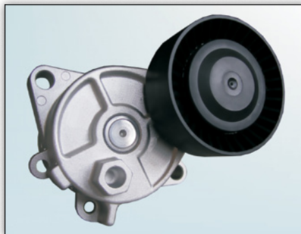
Figura 1: 533 0015 10 (versione meccanica)
