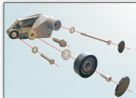
Figura 3: 533 0097 10 - Fornitura
