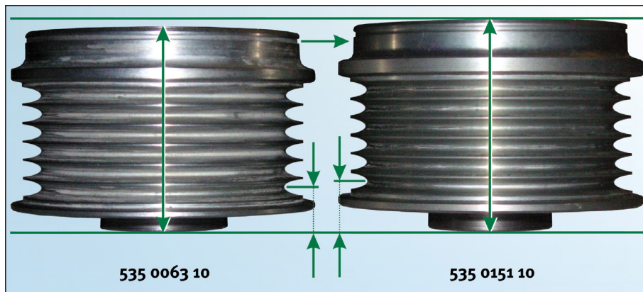
Kuva 3: Laturin vapaapyörien 535 0063 10 (VALEO) ja 535 0151 10 (DENSO) erot.
