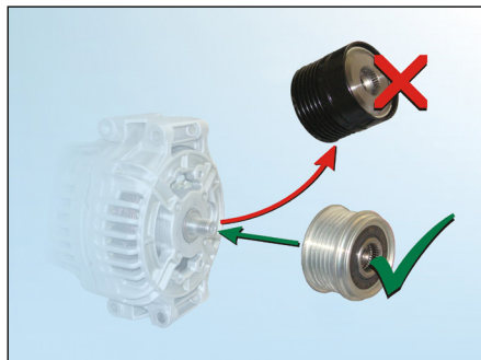
Kuva 1: Alkuperäisosan korvaaminen
