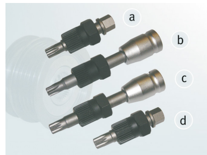
Рис. 2: Обзор специнструмента
