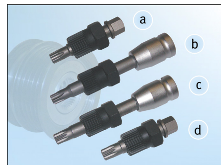
Obrázok 2: Prehľad špeciálneho náradia
