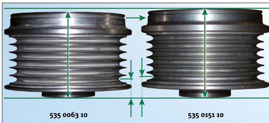
Obrázok 3: Rozlíšenie alternátorových voľnobežiek INA 535 0063 10 (VALEO) a 535 0151 10 (DENSO)
