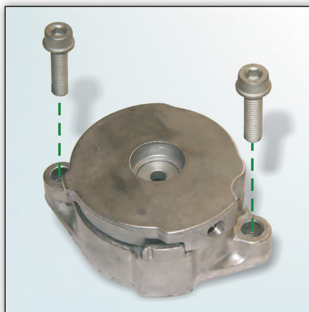
Kuva 1: INA:n kahdella M8x35 ruuvilla varustettu malli
