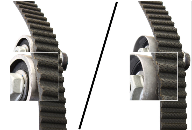
Εικόνα 2: Τροχαλία εκτροπής 532 0623 10 (αριστερά) / τροχαλία εκτροπής 532 0349 10 (δεξιά)
