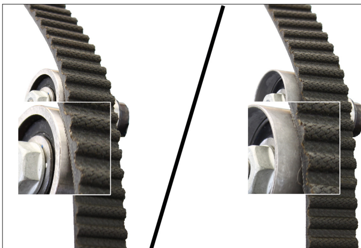
2. ábra: Balra az 532 0623 10 cikkszámú vezetőgörgő/ jobbra az 532 0349 10 cikkszámú vezetőgörgő
