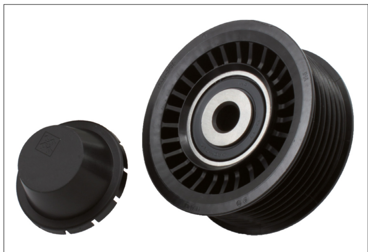
Εικόνα 2: Τροχαλία εκτροπής INA κατασκευασμένη από πλαστικό με καπάκι
