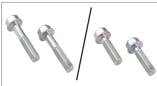
Снимка 4: Ляво, старите M8x40 mm болтове. Дясно, новите M8x30 mm болтове.
