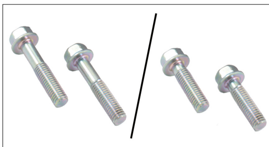
Obrázok 4: Vľavo, staré skrutky M8x40 mm. Vpravo, nové skrutky M8x30 mm.
