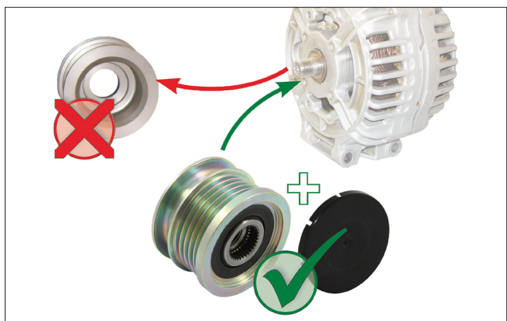
Снимка 1: Промяна от твърда ремъчна ролка към ролка за свободен ход на алтернатор
