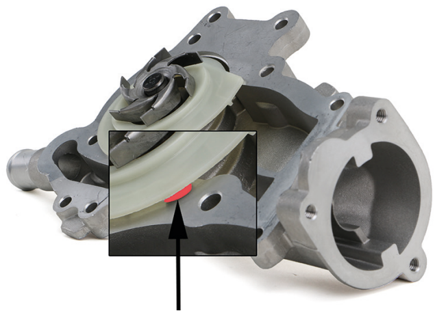
Fig. 2: Loszittende kunststof dichtingsplaat door overtollig afdichtmiddel
