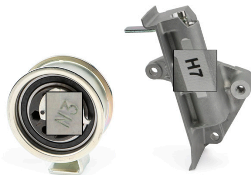
Снимка 1: Обтяжна ролка 531 0396 20 с вибрационен демпфер 533 0039 10
