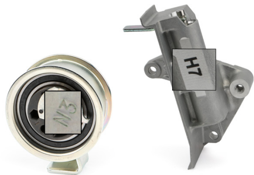
Bild 1: Spannrolle 531 0396 20 mit Schwingungsdämpfer 533 0039 10
