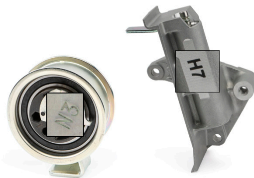
Εικόνα 1: Τεντωτήρας 531 0396 20 με τον αποσβεστήρα 533 0039 10
