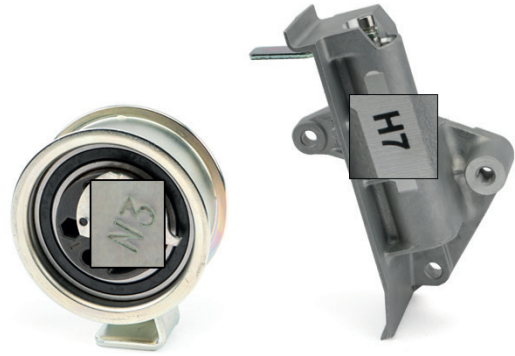
Kuva 1: Kiristinpyörä 531 0396 20 ja värinänvaimennin 533 0039 10
